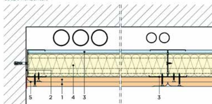
Coupe horizontale
