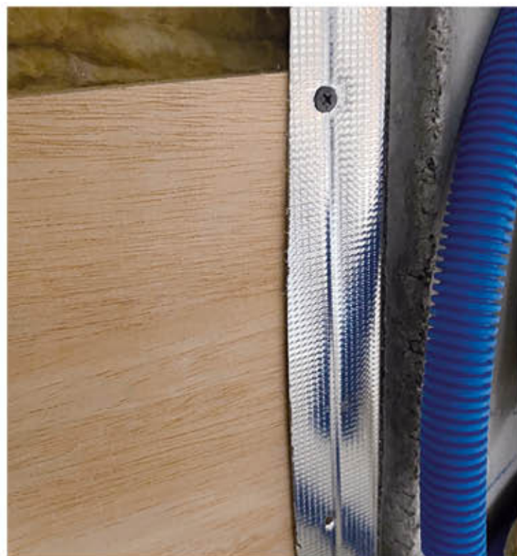
Pose non professionnelle d'une traverse de montage dans la sous-construction.
