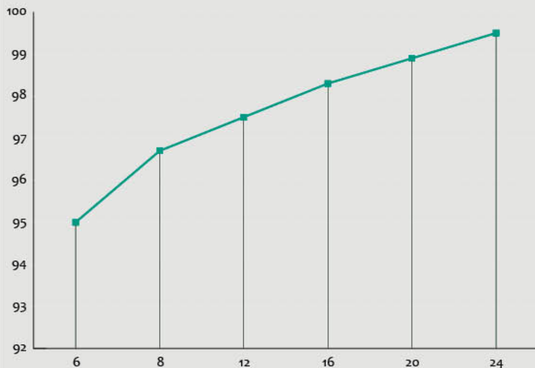
Opacité en fonction % \text{TiO}_2
